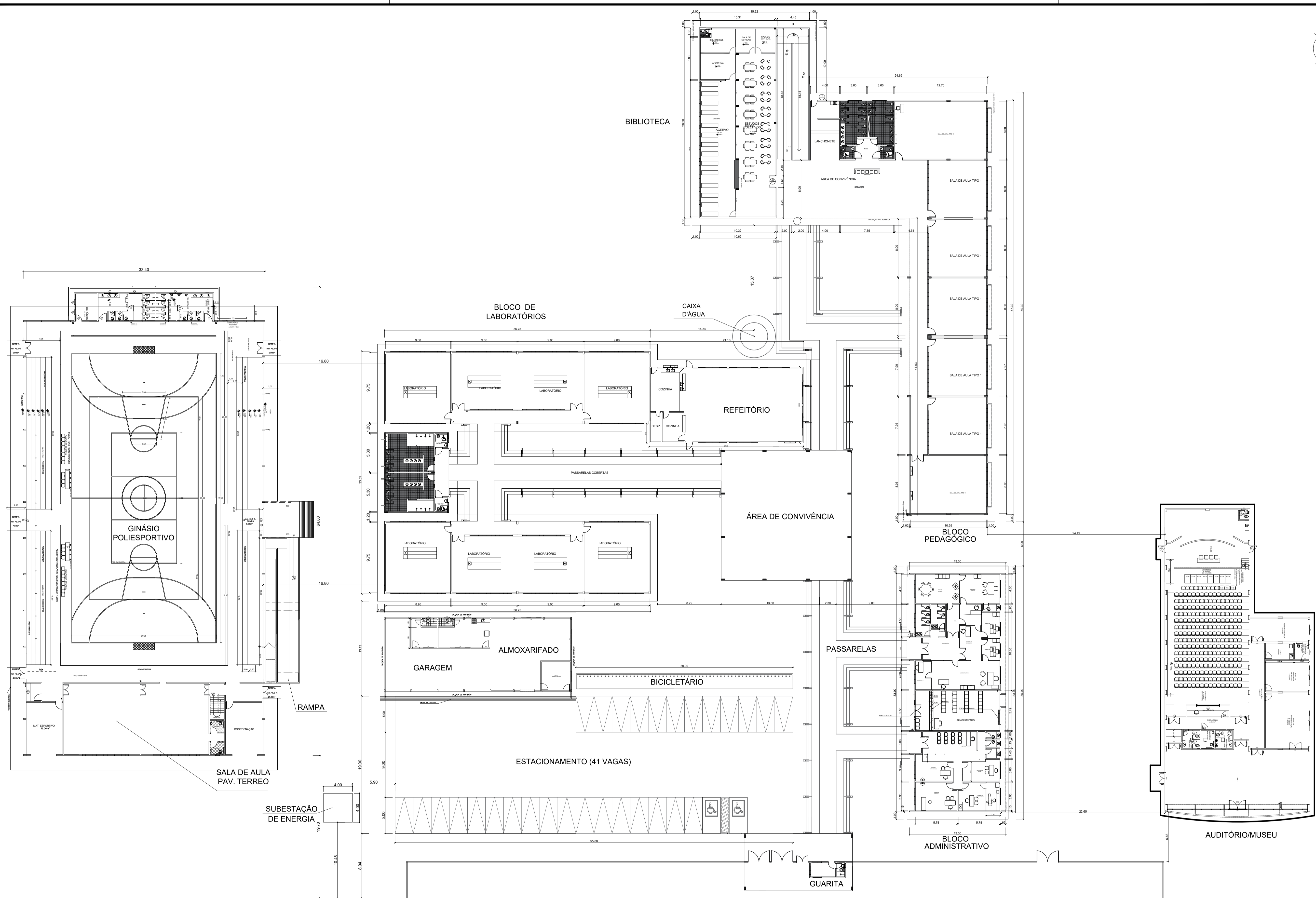
PLANTA DE LOCAÇÃO ESC:1/250
