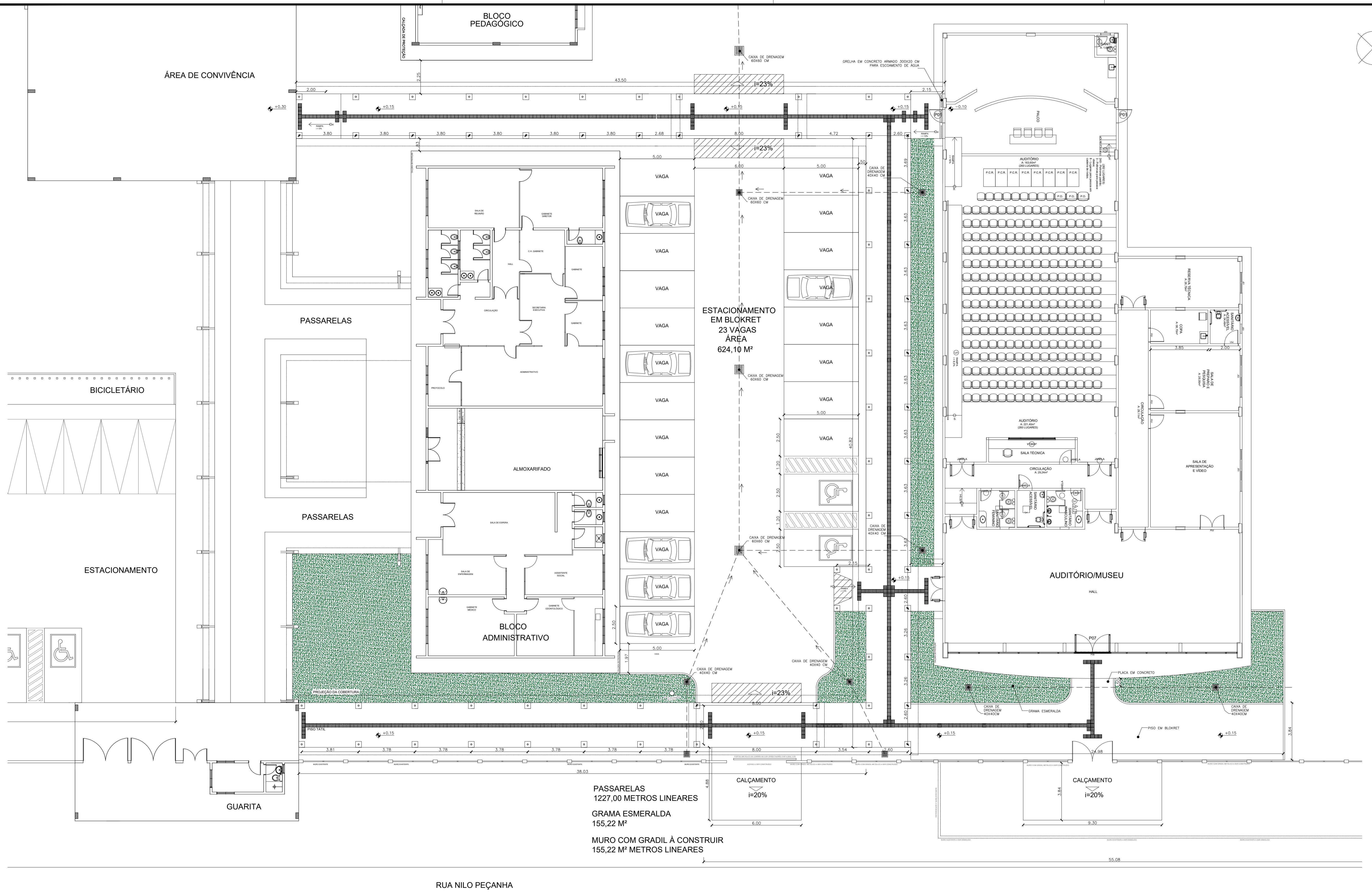
PLANTA DE URBANIZAÇÃO DO ENTORNO DO AUDITÓRIO ESC:1/120
